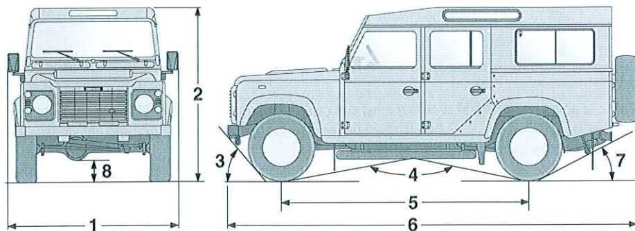
Dimensions du Station Wagon 110
